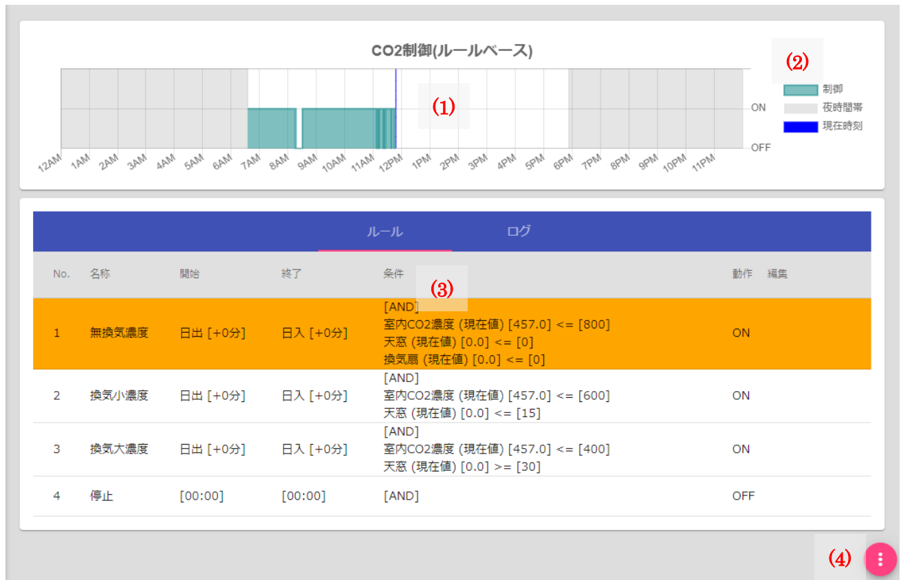
図 27：ルールベース制御モニター画面
