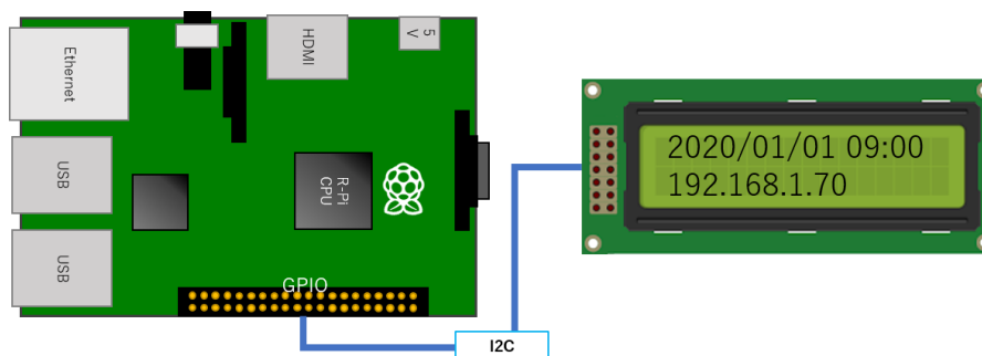
図 52：LCD デバイス接続模式図
