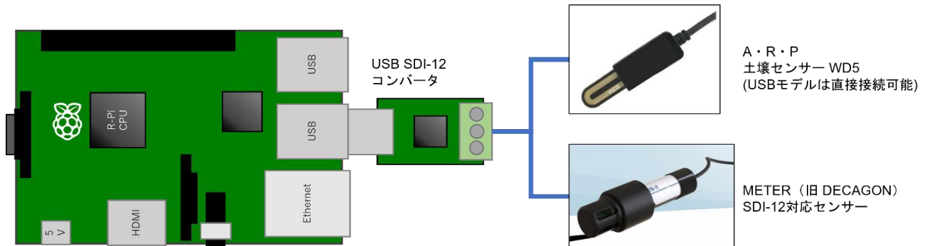
図 50 : SDI-12 デバイス接続模式図
