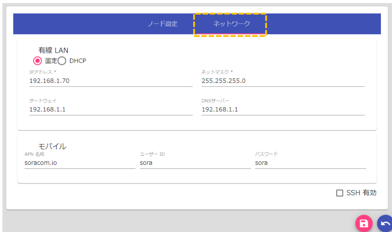
図 64：ネットワーク設定画面
