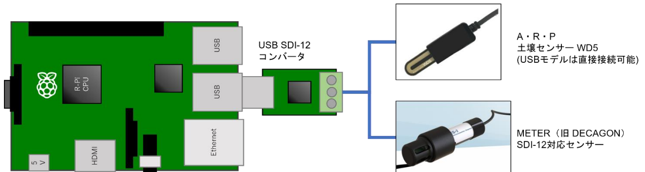
図 56 : SDI-12 デバイス接続模式図
