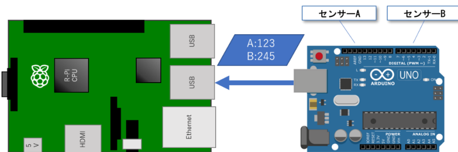
図 54：汎用シリアル入力デバイス接続模式図
