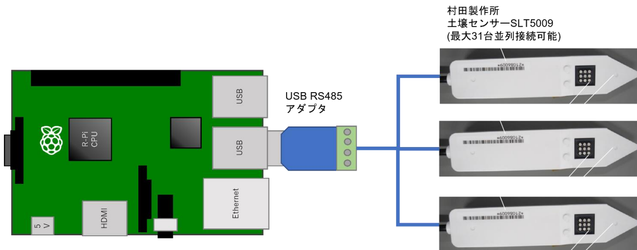
図 45 : SLT5009 接続模式図
