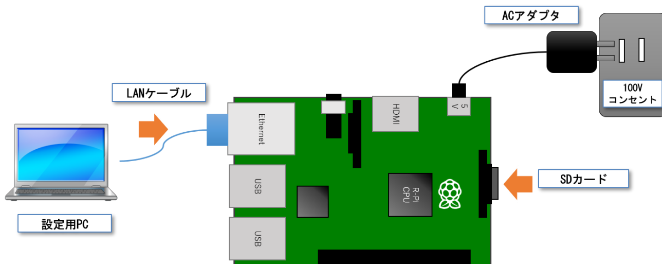
図 3：設定用 PC 接続モード図
