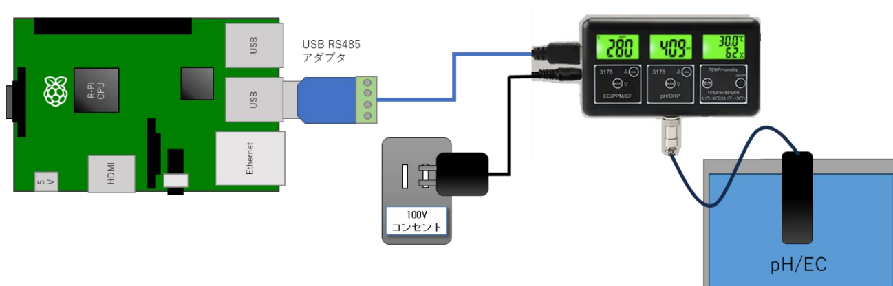
図 50：水質センサー接続模式図
