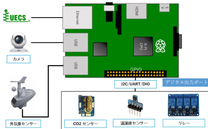
図 40：デバイス接続模式図
