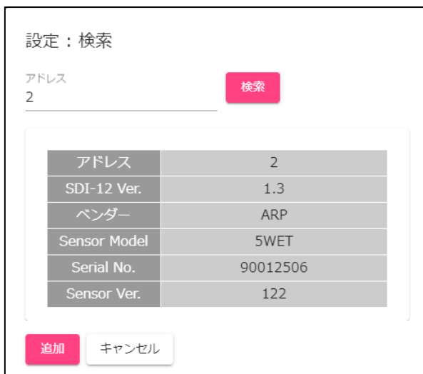
[デバイス追加ダイアログ]
