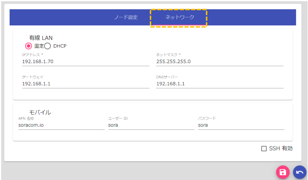
図 70：ネットワーク設定画面
