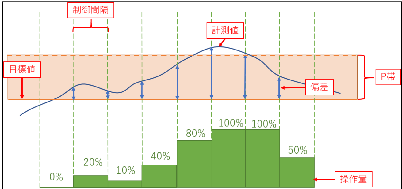
図 32 : P 比例動作イメージ
