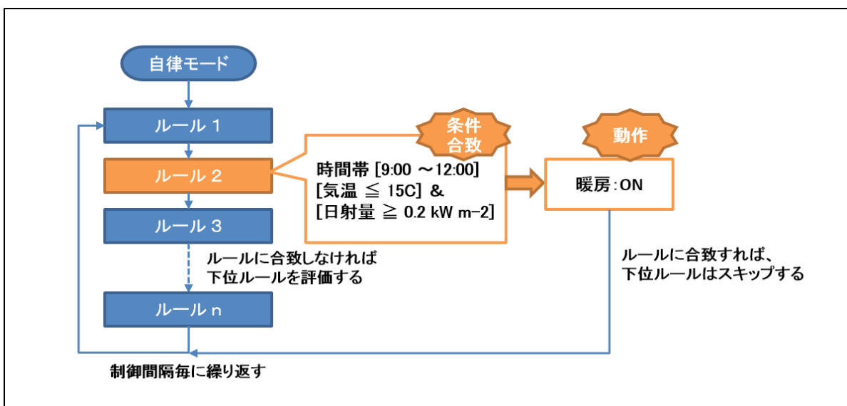
図 26：ルールベース制御概念図
