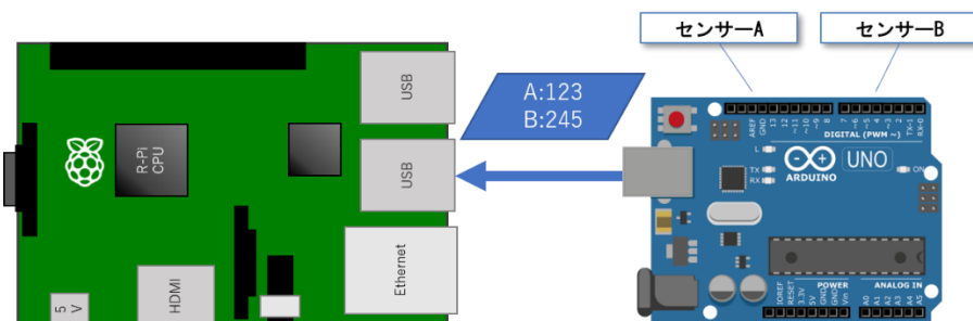
図 47：汎用シリアル入力デバイス接続模式図
