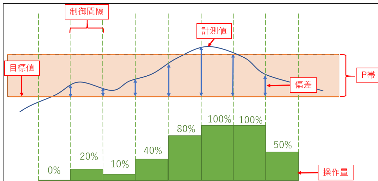
図 31 : P 比例動作イメージ
