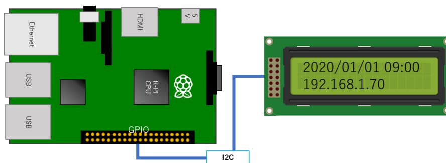
図 49 : LCD デバイス接続模式図
